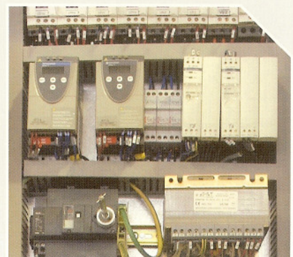
Quadro elettrico Tableau électrique
