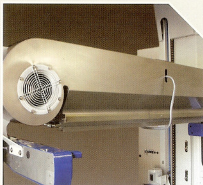
Asciugatura a seguire il profilo del veicolo Séchage à suivre le profil du véhicule
